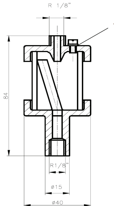
Bild 1 - Rücklaufsicherung ZG 4.1.
