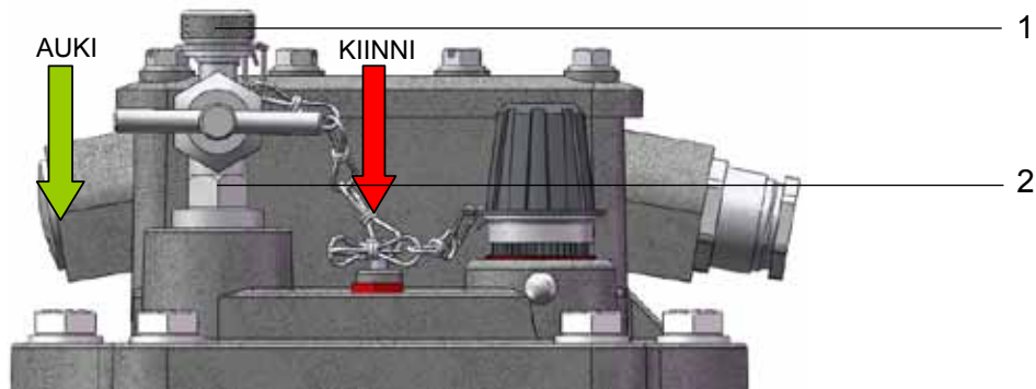
Kuva 2 - Ilmanpoistoveniili
